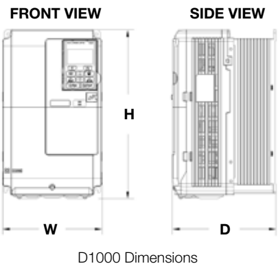
D1000 Dimensions
